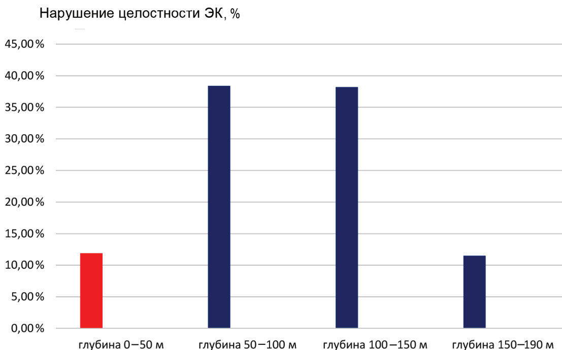
Рис. 6. Диаграмма распределения нарушений целостности из труб ПНД 110×18 по глубине скважин / Fig. 6. Diagram of the integrity violations distribution from HDPE pipes 110×18 by the depth of wells
